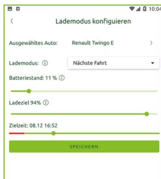
113 App: Bildschirm "Lademodus konfigurieren"
