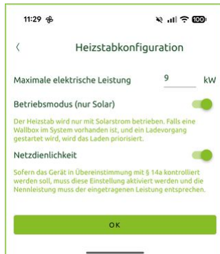
51 App: Bildschirm "Heizstabkonfiguration"
