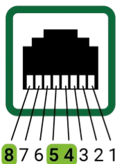
14 RJ45 Pinbelegung ab SN 1000
