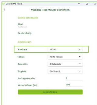
59 App: Bildschirm "Modbus-RTU Einstellungen"
