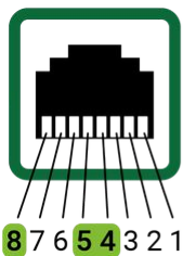
13 RJ45 Pinbelegung bis SN 1000
