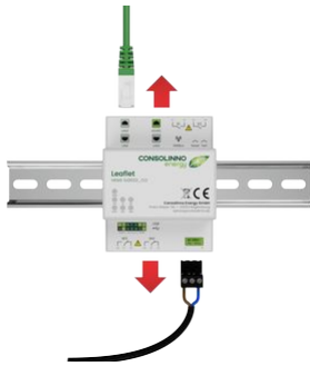
135 Demontage 3: Verkabelung lösen
