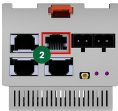
12 RS485 Schnittstelle
