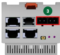
16 Schließer-Relais-Anschlüsse
