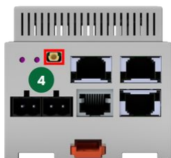
23 wM-Bus Antennenanschluss
