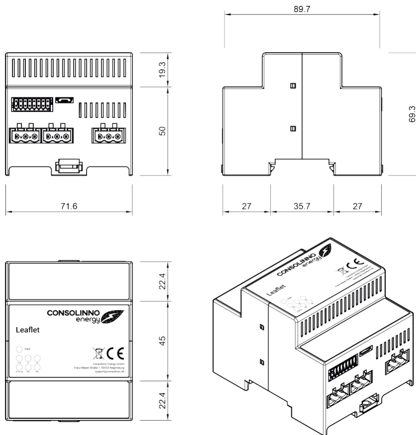
137 Abmessungen des Consolinno Leaflet HEMS
