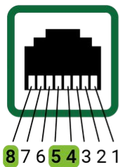
14 RJ45 Pinbelegung bis SN 1000
