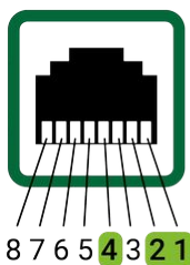
15 RJ45 Pinbelegung ab SN 1000
