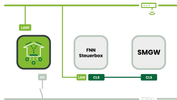
85 Verbindung mit der FNN Steuerbox über EEBus
