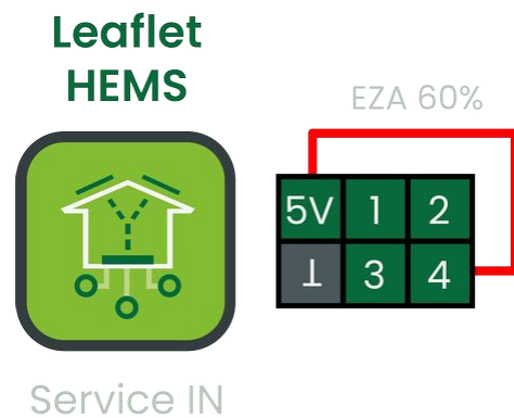
84 60% Dimmung OHNE ImSys und Steuerbox
