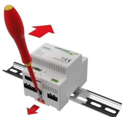
151 Demontage 4: Gerät von der Hutschiene nehmen
