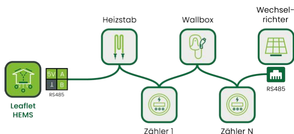
16 Schematische Darstellung einer Daisy-Chain-Verkabelung (Beispiel)
