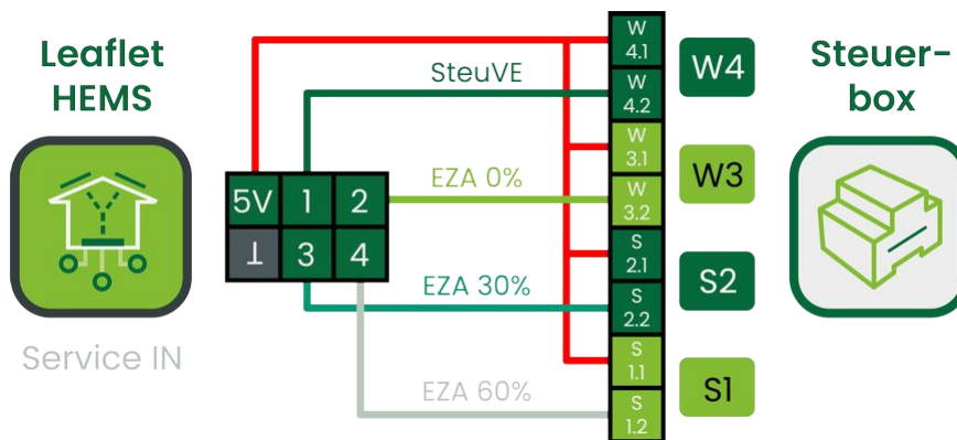
72 Relaisverbindung LPP §9 und LPC §14a
