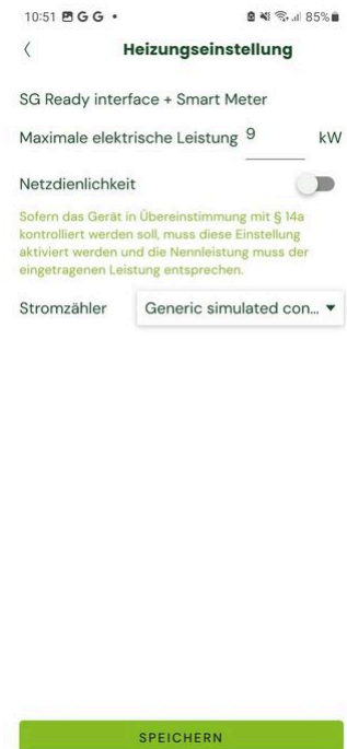
124 App: Bildschirm "SG Ready Zähler"
