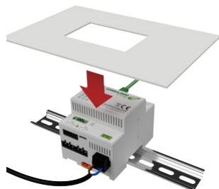
8 Einbau 3: Abdeckung anbringen
