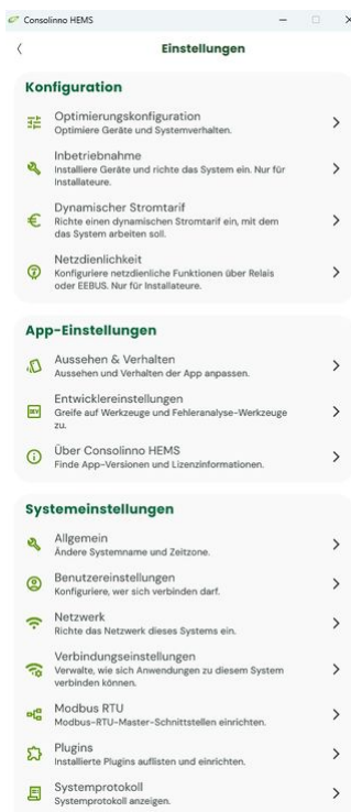
75 App: Bildschirm "Einstellungen"
