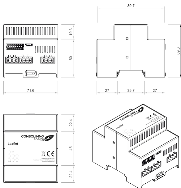
137 Abmessungen des Consolinno Leaflet HEMS
