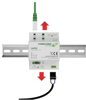
135 Demontage 3: Verkabelung lösen
