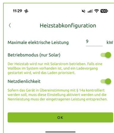
128 App: Bildschirm "Heizstabkonfiguration"
